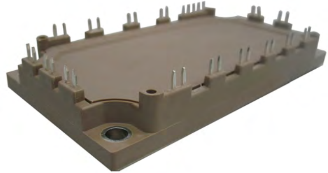
Rectifier+Brake+Inverter
